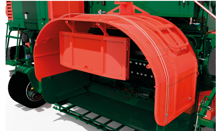
Prolongación de capot plegada en posición de transporte.
